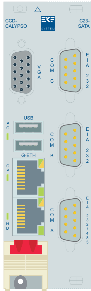
CCD-CALYPSO w. C23-SATA © EKF ekf.com VGA Video Option
