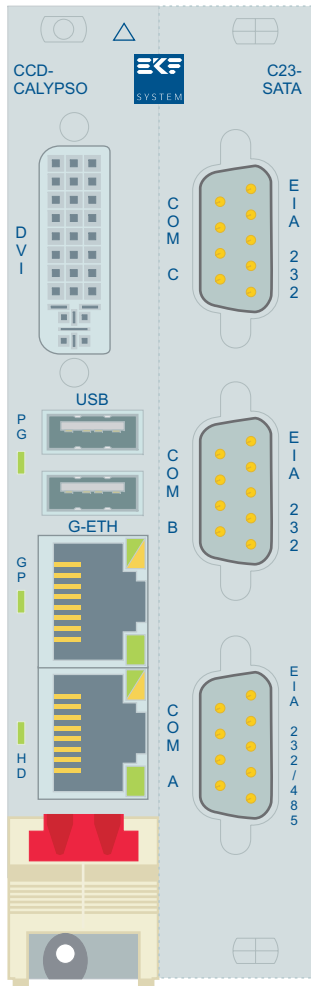
CCD-CALYPSO w. C23-SATA © EKF ekf.com DVI-I Video Option
