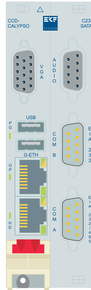
CCD-CALYPSO w. C23-SATA © EKF ekf.com VGA & Audio Option
