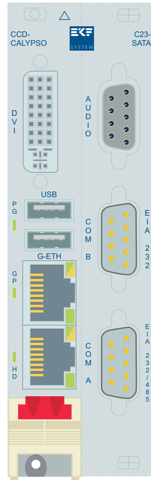
CCD-CALYPSO w. C23-SATA © EKF ekf.com DVI-I & Audio Option
